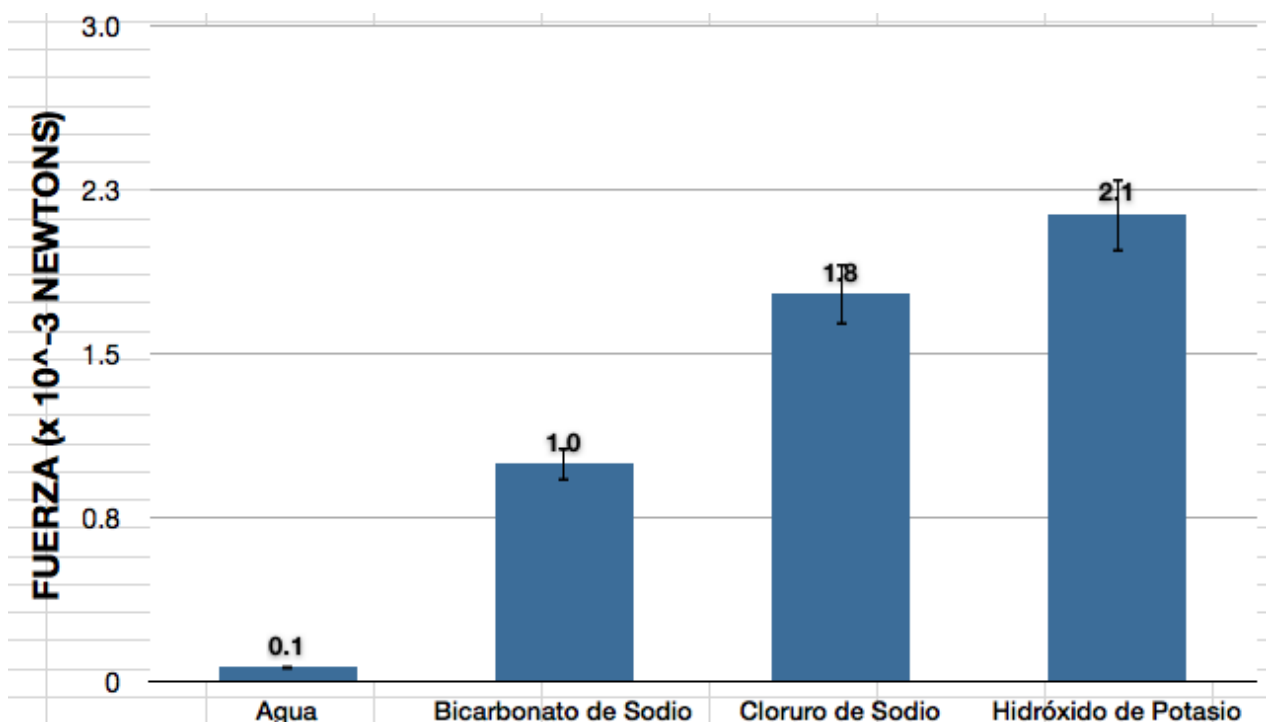
Fig. 6 Fuerzas obtenidas. Se utilizó la fórmula F = I \times B con los valores de las intensidades que se obtuvieron como se indica en la figura 5 y el valor del campo magnético (0.3 Teslas).
